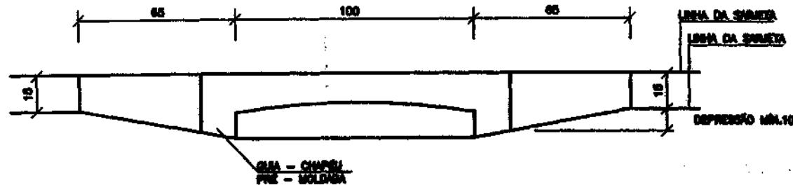
CORTE AA'
