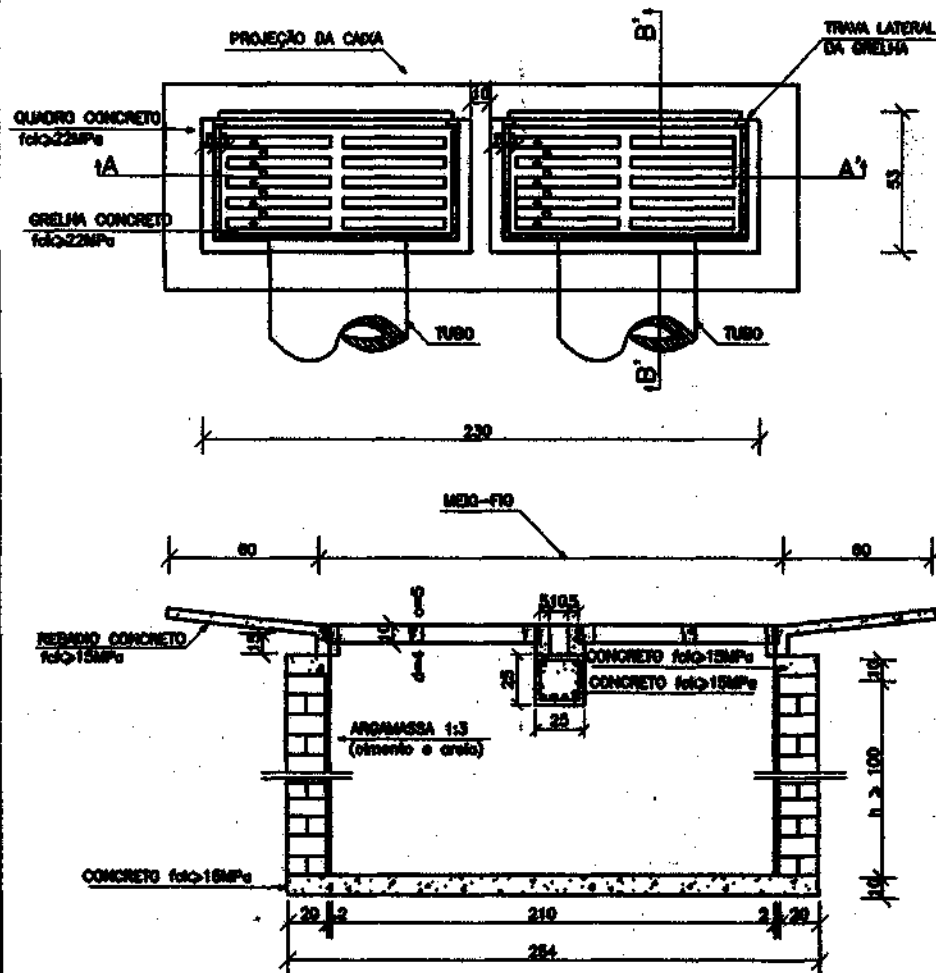
PLANTA
