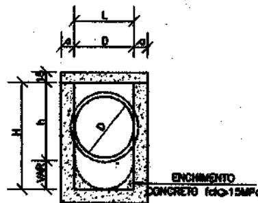
CORTE BB'
